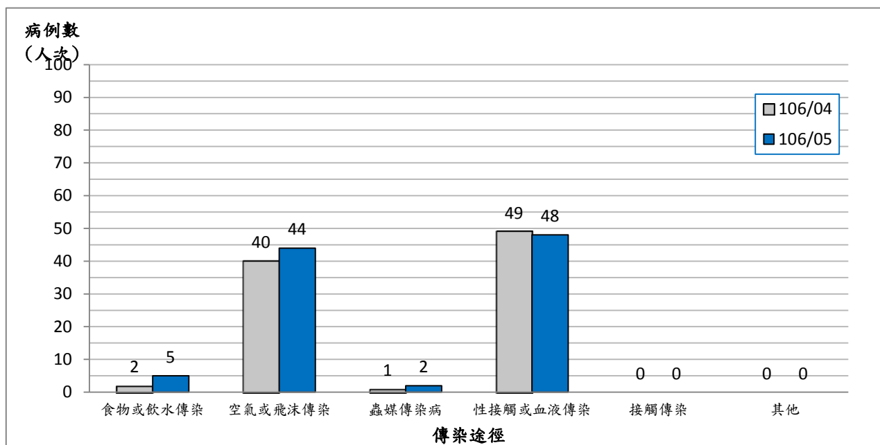
圖2. 彰化縣各類傳染病傳染途徑病例數(106年4月底v.s.106年5月底)
