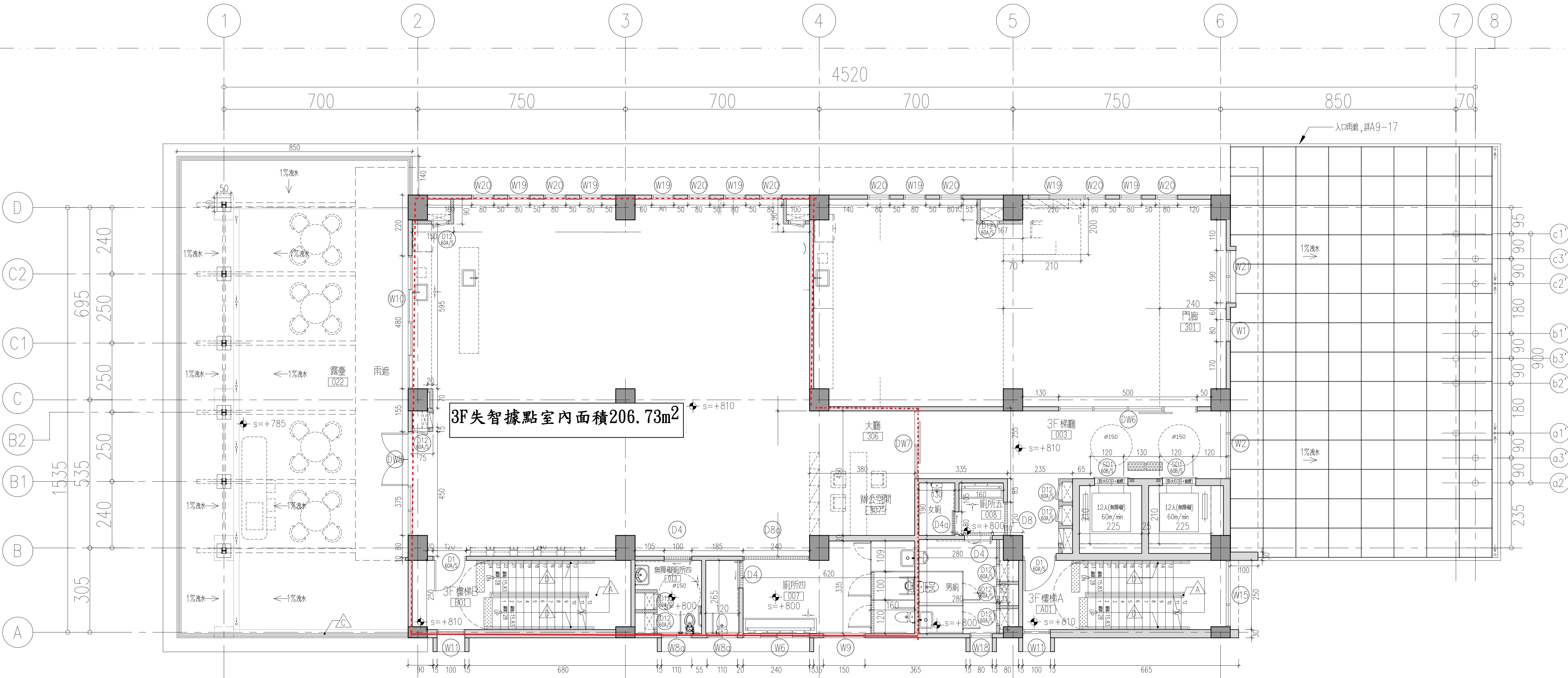
1 三層平面圖
